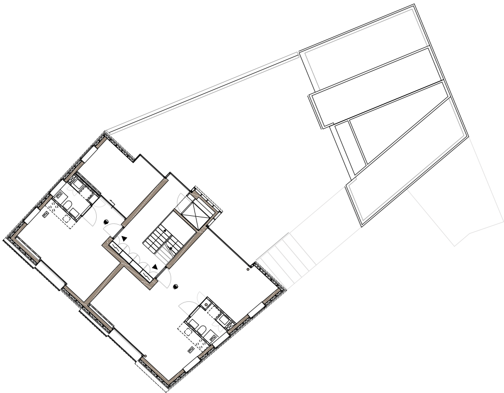
Vierde verdieping
