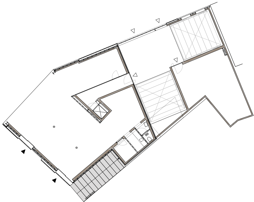
Begane grond
