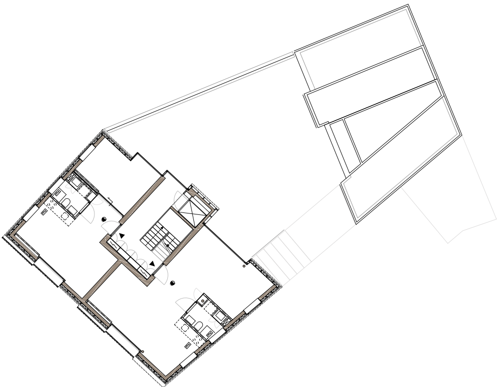
Derde verdieping
