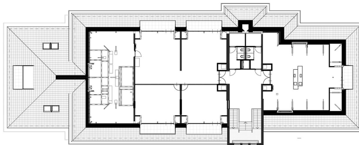
plattegrond +2
