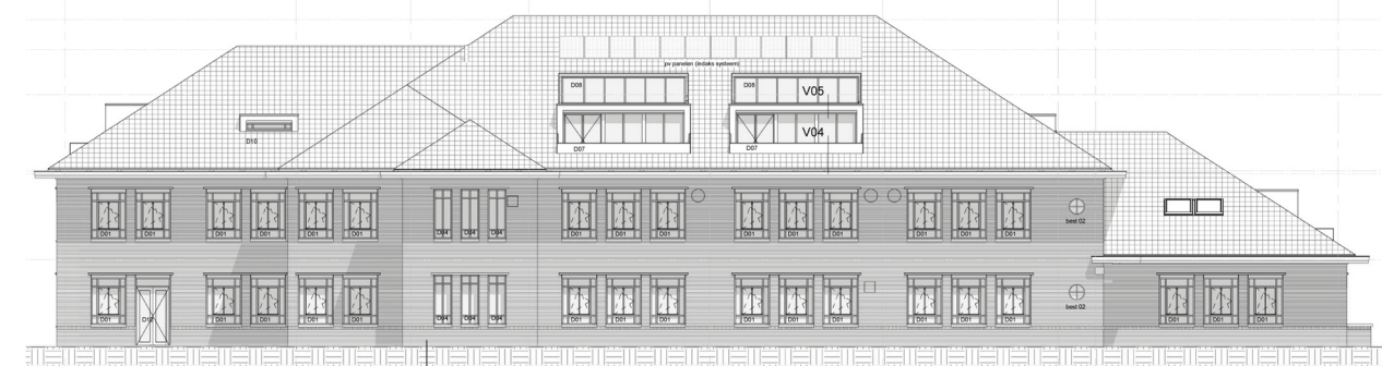
achtergevel
