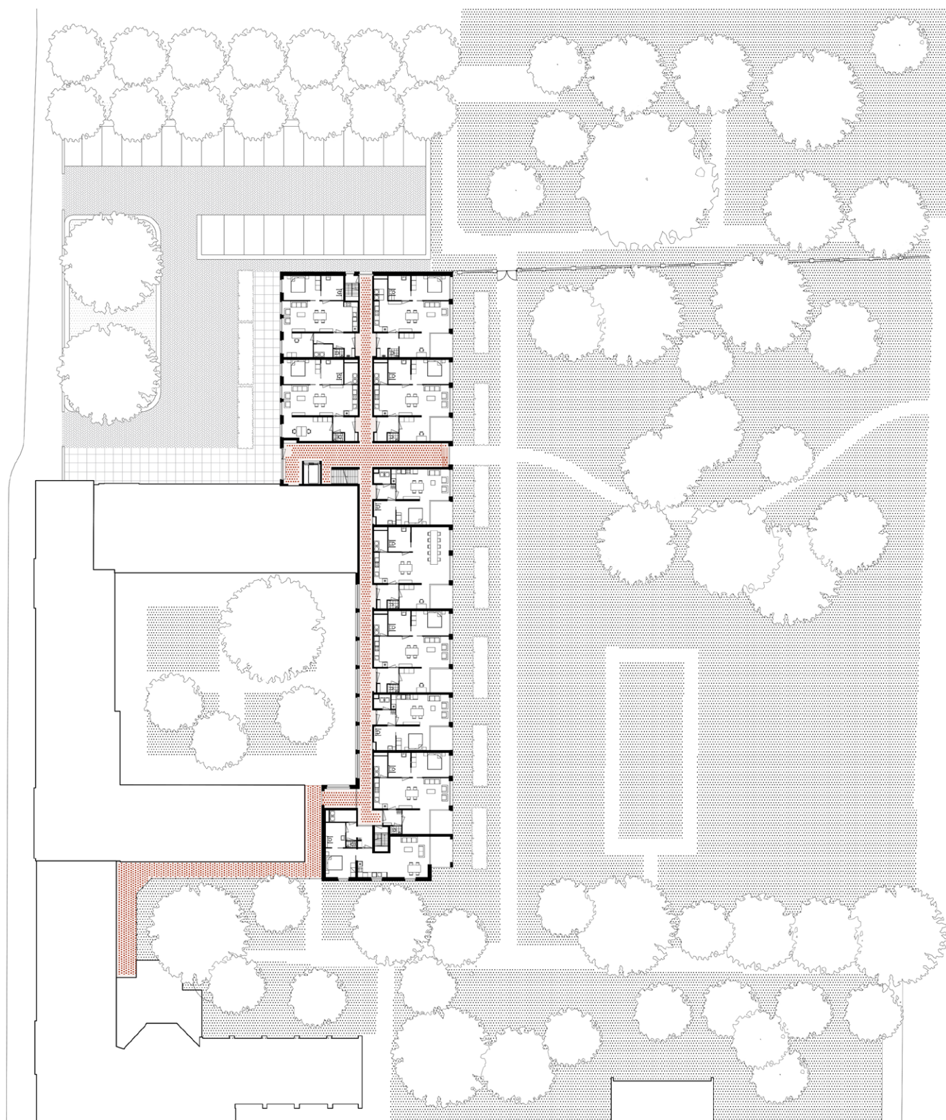
plattegrond woongebouw fase 1
