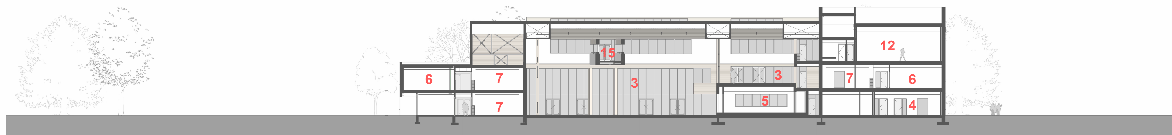
Doorsnede B
