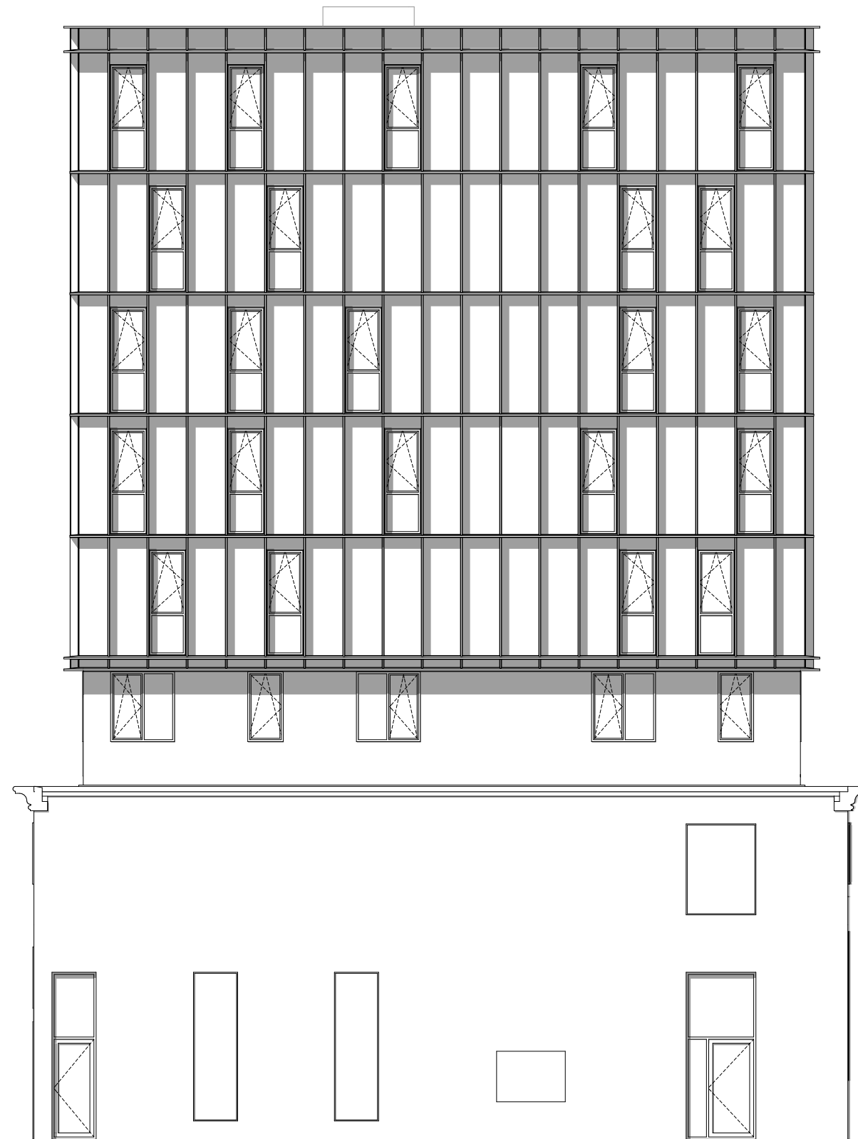
WESTGEVEL
