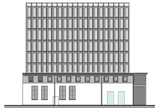
verdeling gevel vijfdeling per stramien
