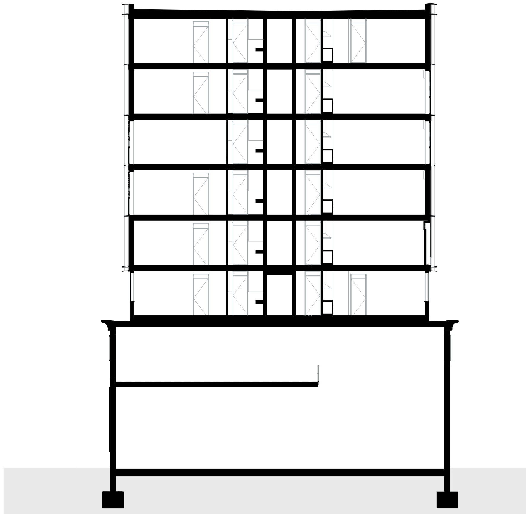
DOORSNEDE
