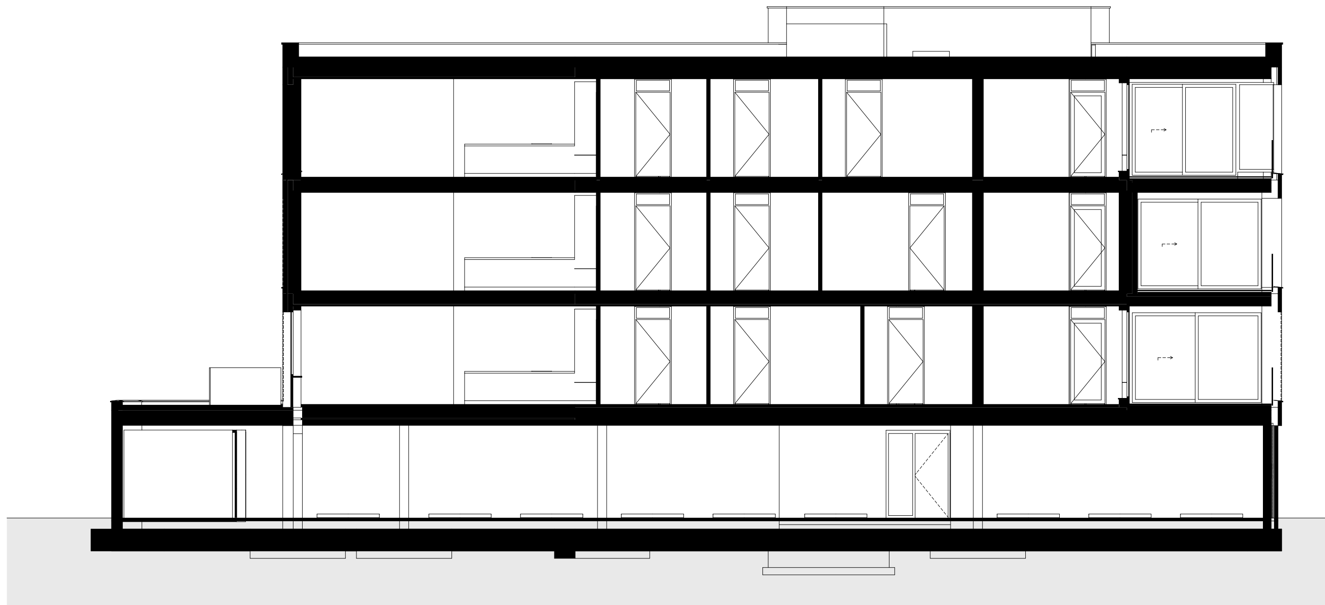
DOORSNEDE A-A
