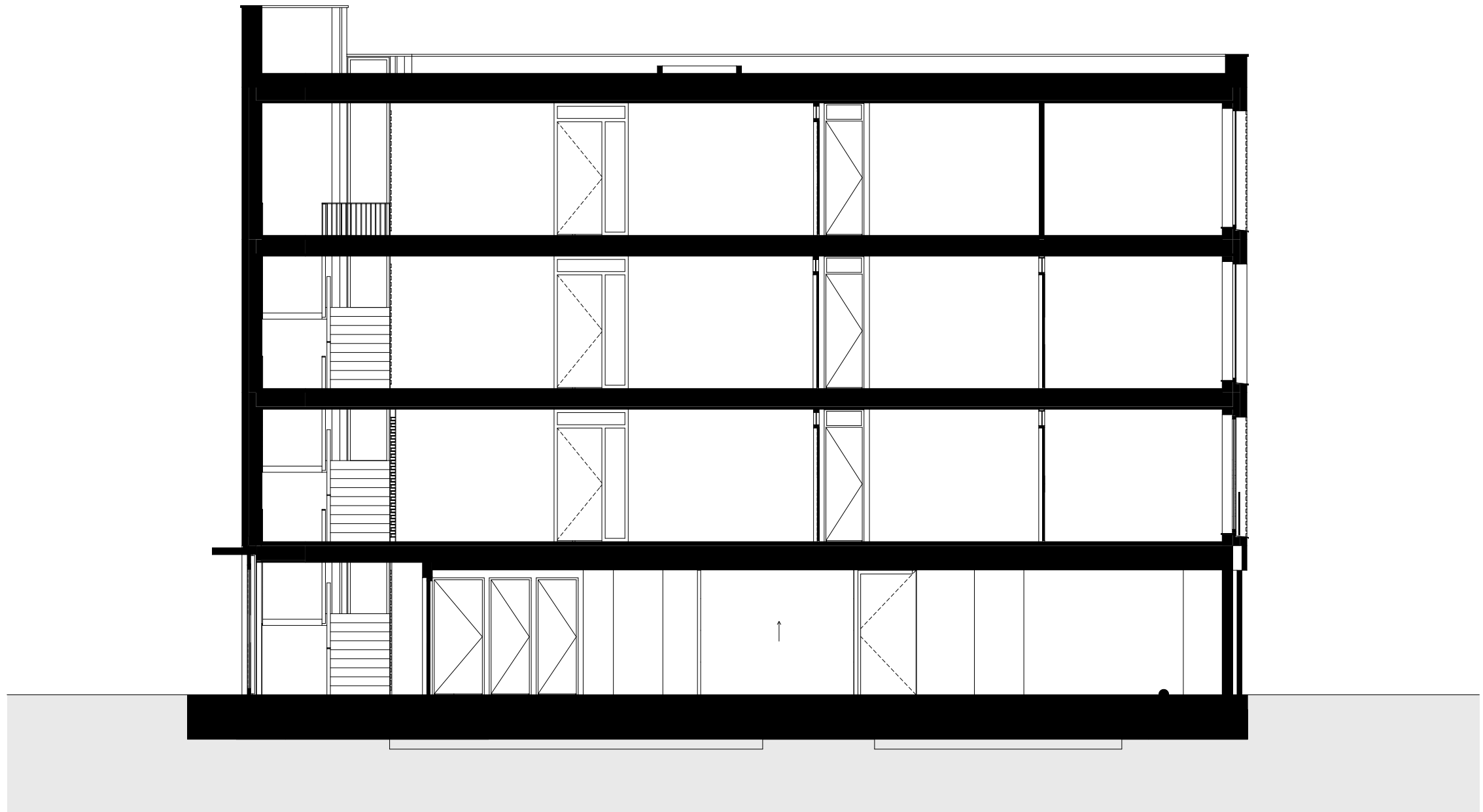
DOORSNEDE B-B
