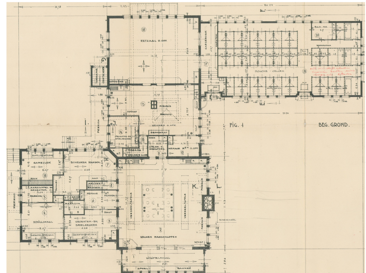
plattegrond begane grond 1938
