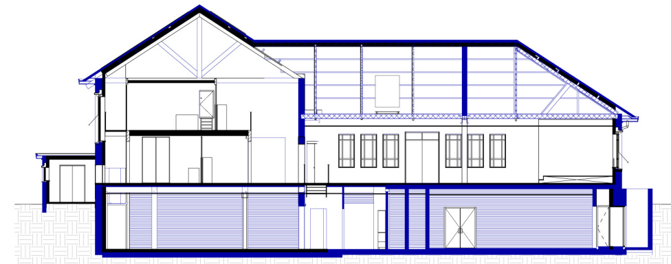
doorsnede A
