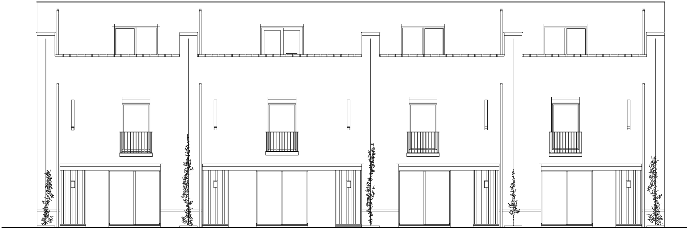
gevel B | schaal 1:100
