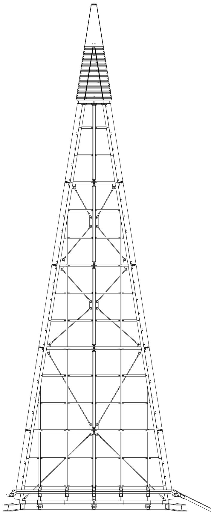
vooraanzicht
