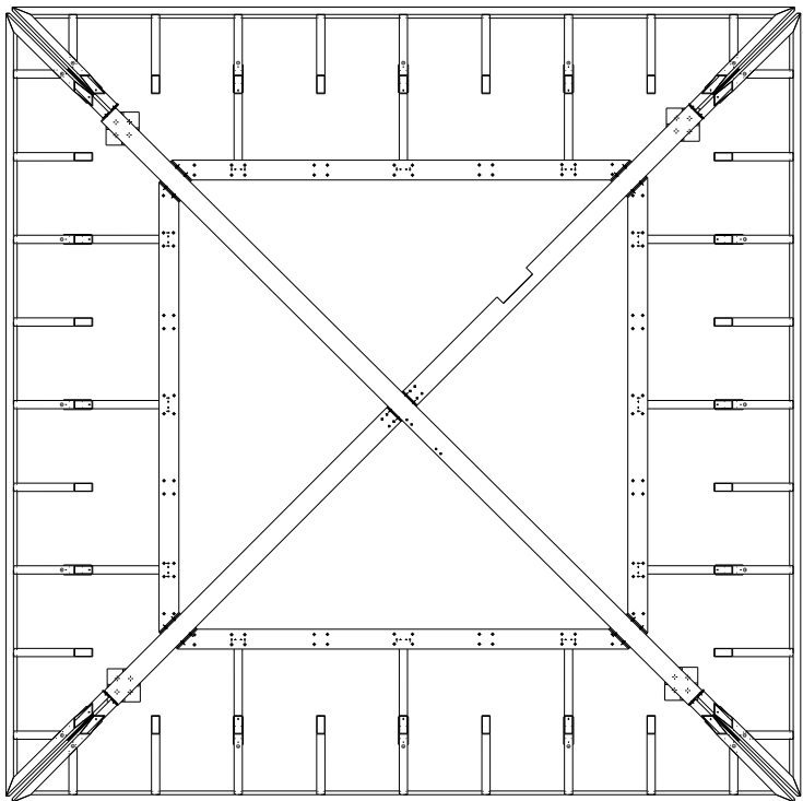
bovenaanzicht onderframe
