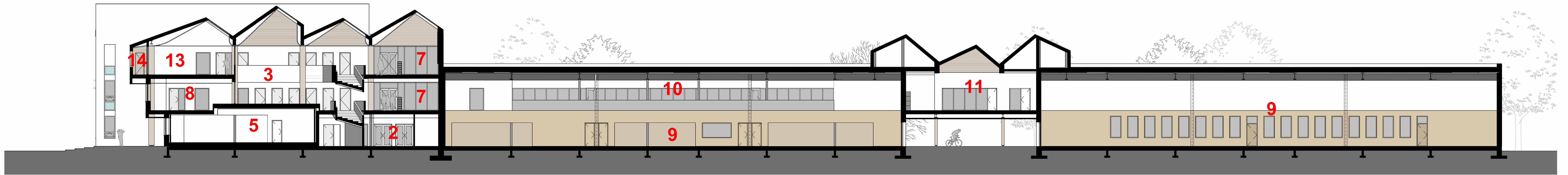
Doorsnede A
