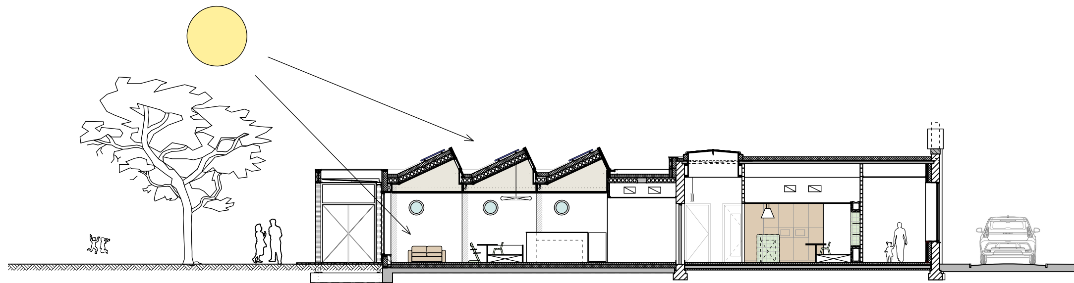
dwarsdoorsnede
